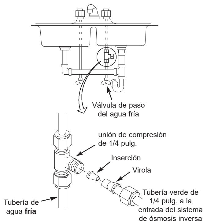
Conexión de suministro de agua fría (con la unión de compresión - no se incluye)
