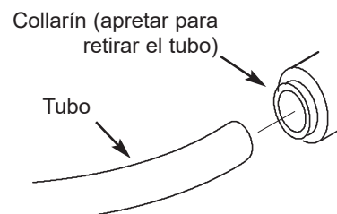
Desconecte el tubo
